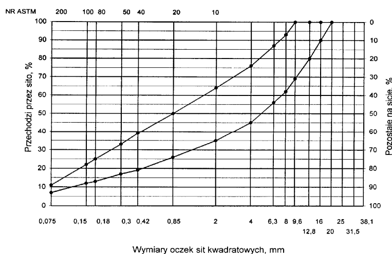
Rys. 1. Krzywe graniczne uziarnienia mieszanki min. BA od 0 do 20 mm do w-wy ścieralnej nawierzchni drogi o
