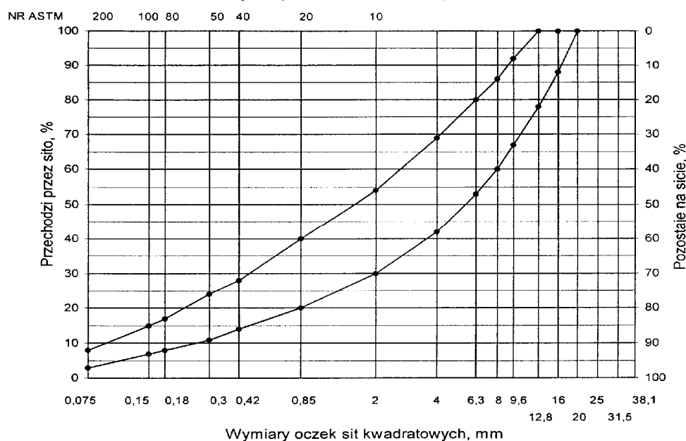
Rys. 8. Krzywe graniczne uziarnienia mieszanki mineralnej BA od 0 do 20 mm do warstwy wiążącej, wyrównawczej i wzmacniającej nawierzchni drogi o obciążeniu ruchem KR1 lub KR2 Rys. 9. Krzywe graniczne uziarnienia mieszanki
