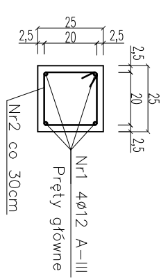
Szczegóły wieńca W-1 skala 1:20
