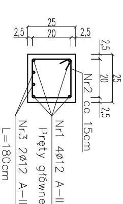
Szczegóły nadproża W-1.1 skala 1:20
