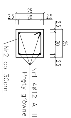
Szczegóły wieńca R-1 skala 1:20
