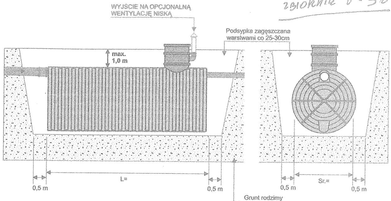
Rysunek 2. Posadowienie zbiornika z polietylenu ( grunt gliniasty, ilasty, możliwość występowania wód gruntowych )
