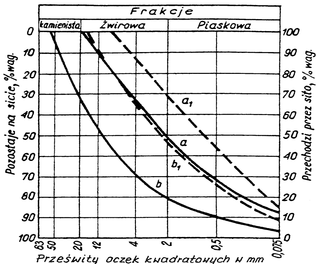
Rysunek 1. Obszar uziarnienia optymalnych mieszanek żwirowych
