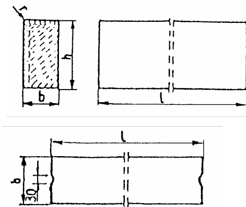
Rys. 1. Wymiarowanie krawężników
