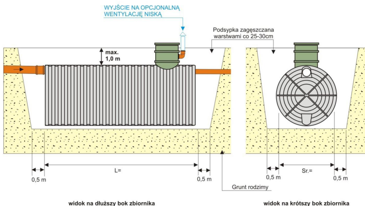
Rysunek 1. Posadowienie zbiornika z polietylenu ( grunt piaszczysty, woda gruntowa nie występuje )
