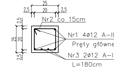
Szczegóły nadproża W-1.1 skala 1:20
