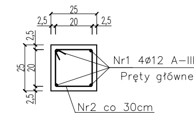
Szczegóły wieńca W-1 skala 1:20
