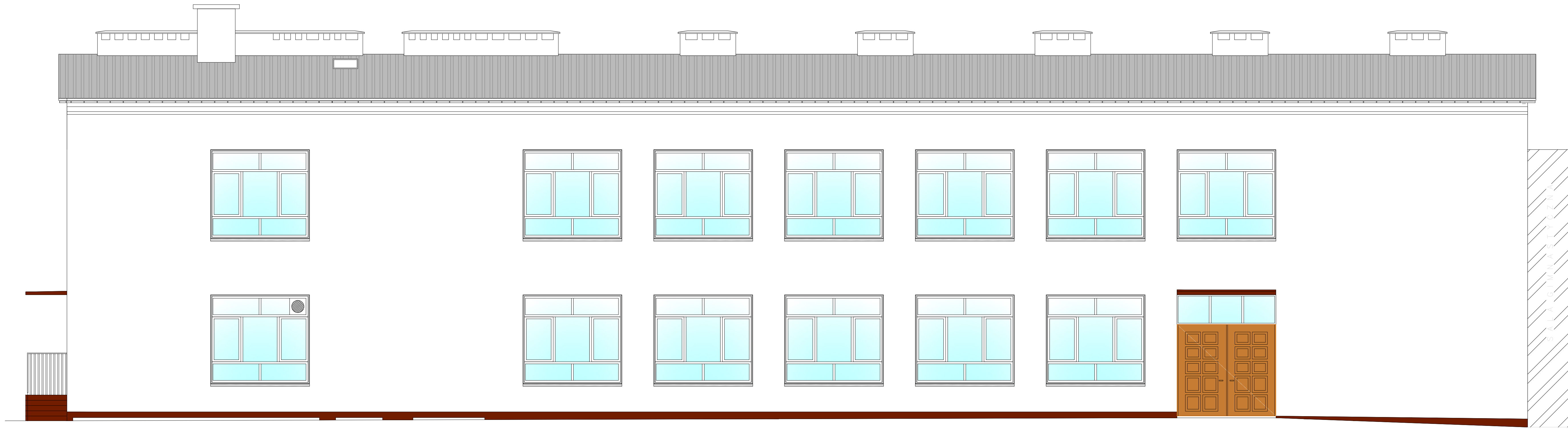
ELEWACJA PÓŁNOCNO–ZACHODNIA Skala 1:100
