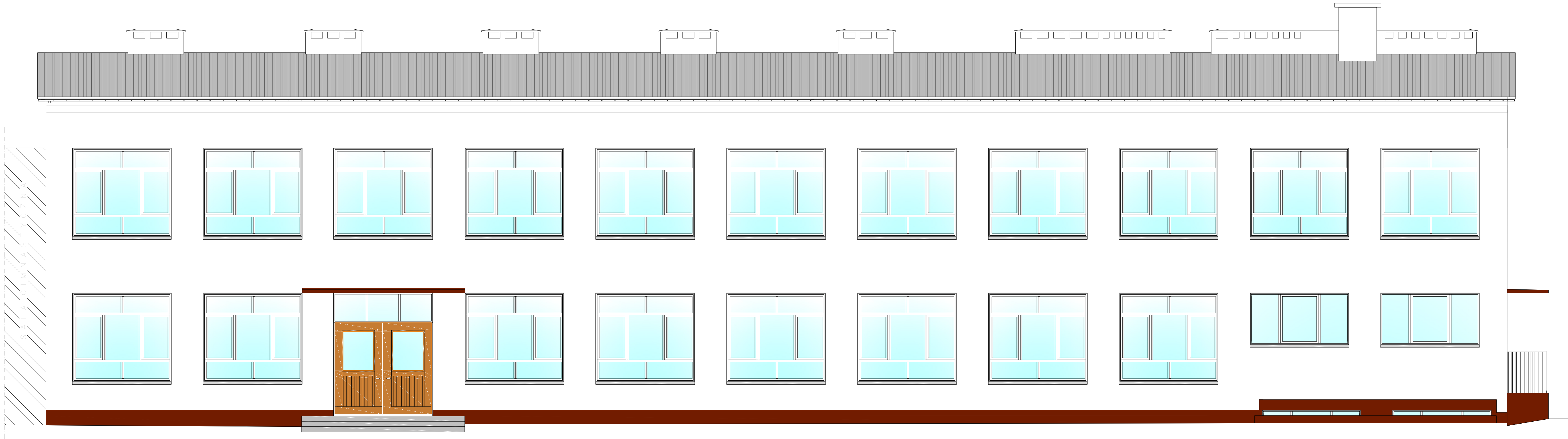
ELEWACJA POŁUDNIOWO–WSCHODNIA Skala 1:100
