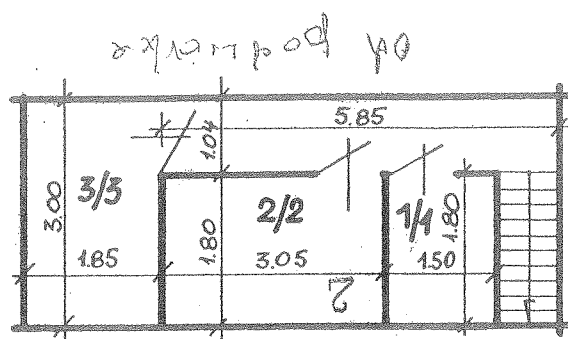
RZUT PIWNIC
