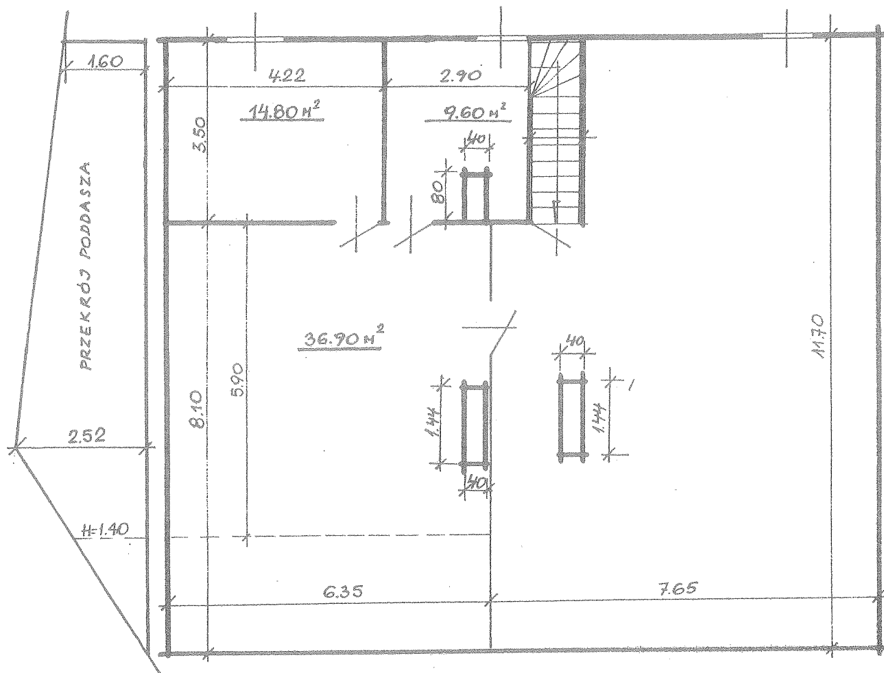
RZUT PODDASZA
