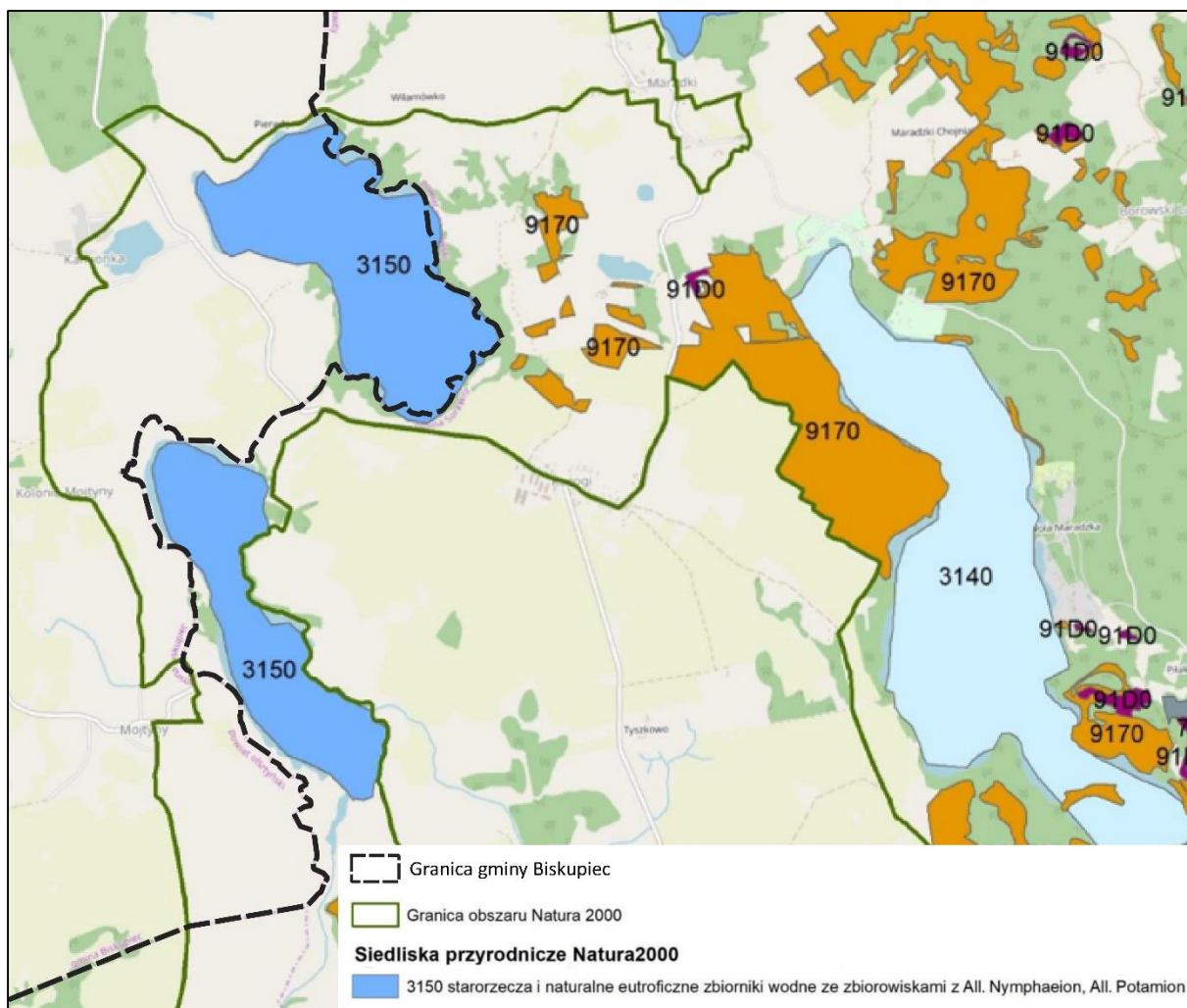
Ryc. 21 Cenne siedliska przyrodnicze Obszaru Natura 2000 Ostoja Piska PLH280048 występujące bezpośrednio na terenie gminy Biskupiec
