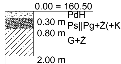
Profil odwiertu nr G4
