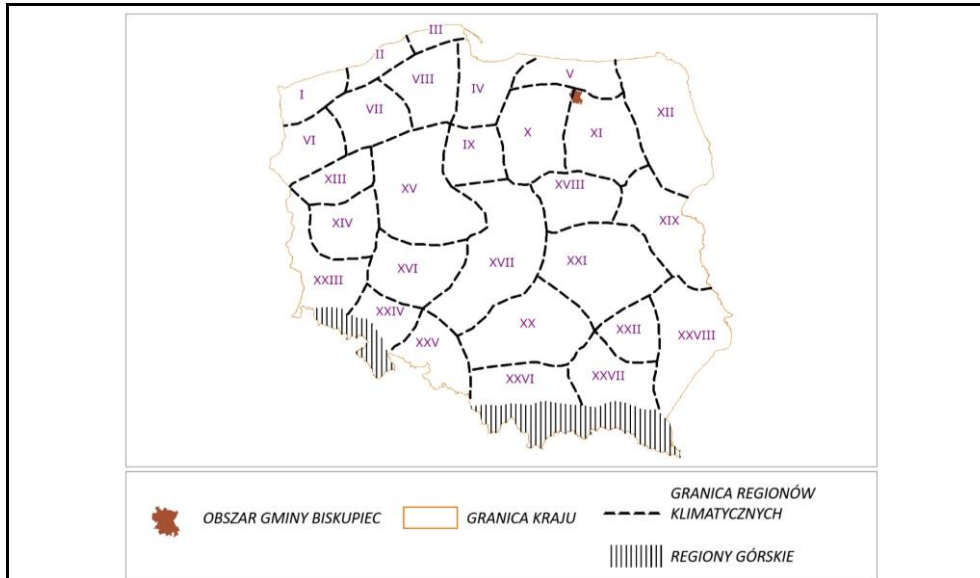
Rycina 5 Położenie gminy Biskupiec na tle regionalizacji klimatycznej Polski
