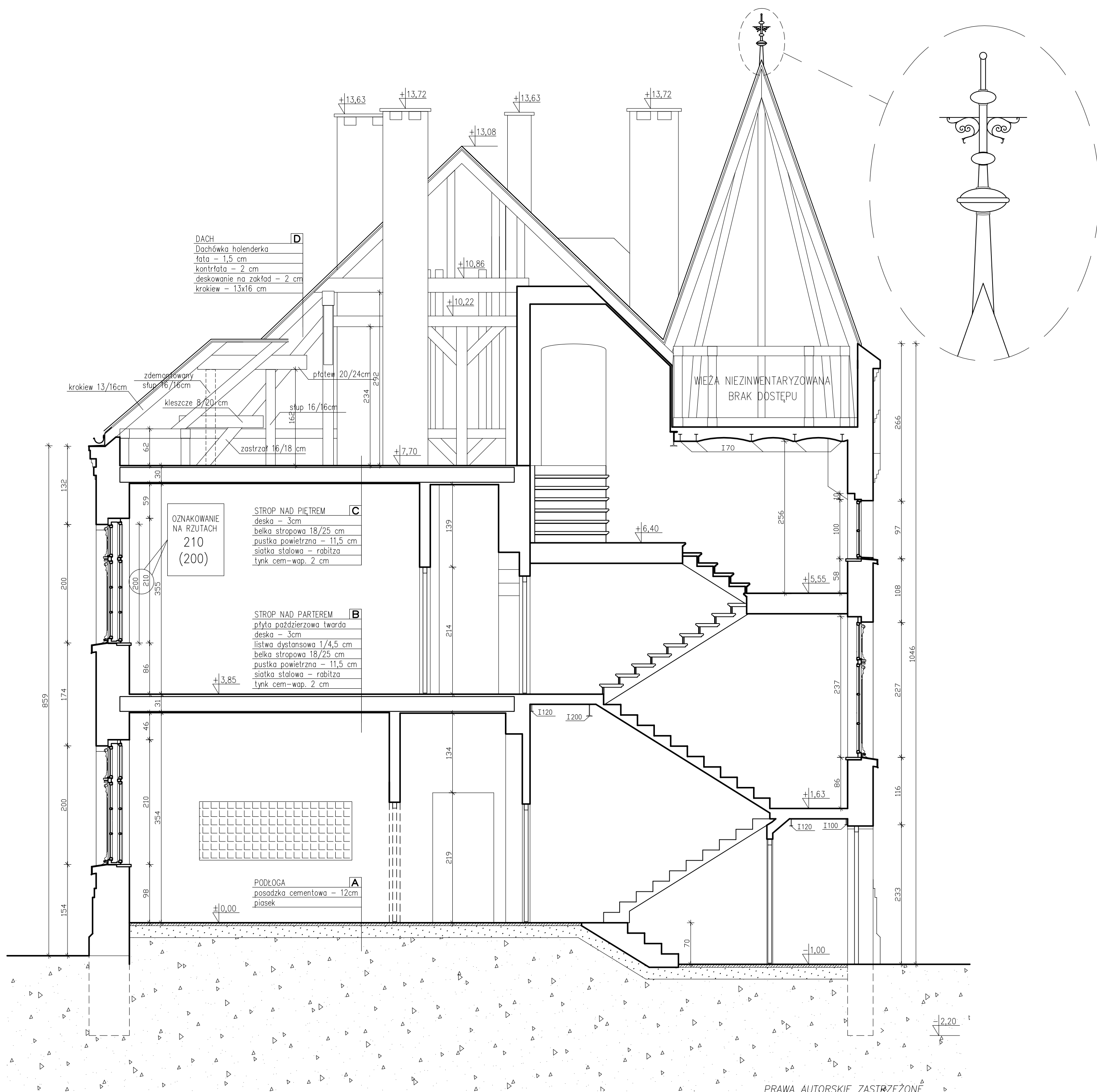
PRZEKRÓJ A-A SKALA 1:50
