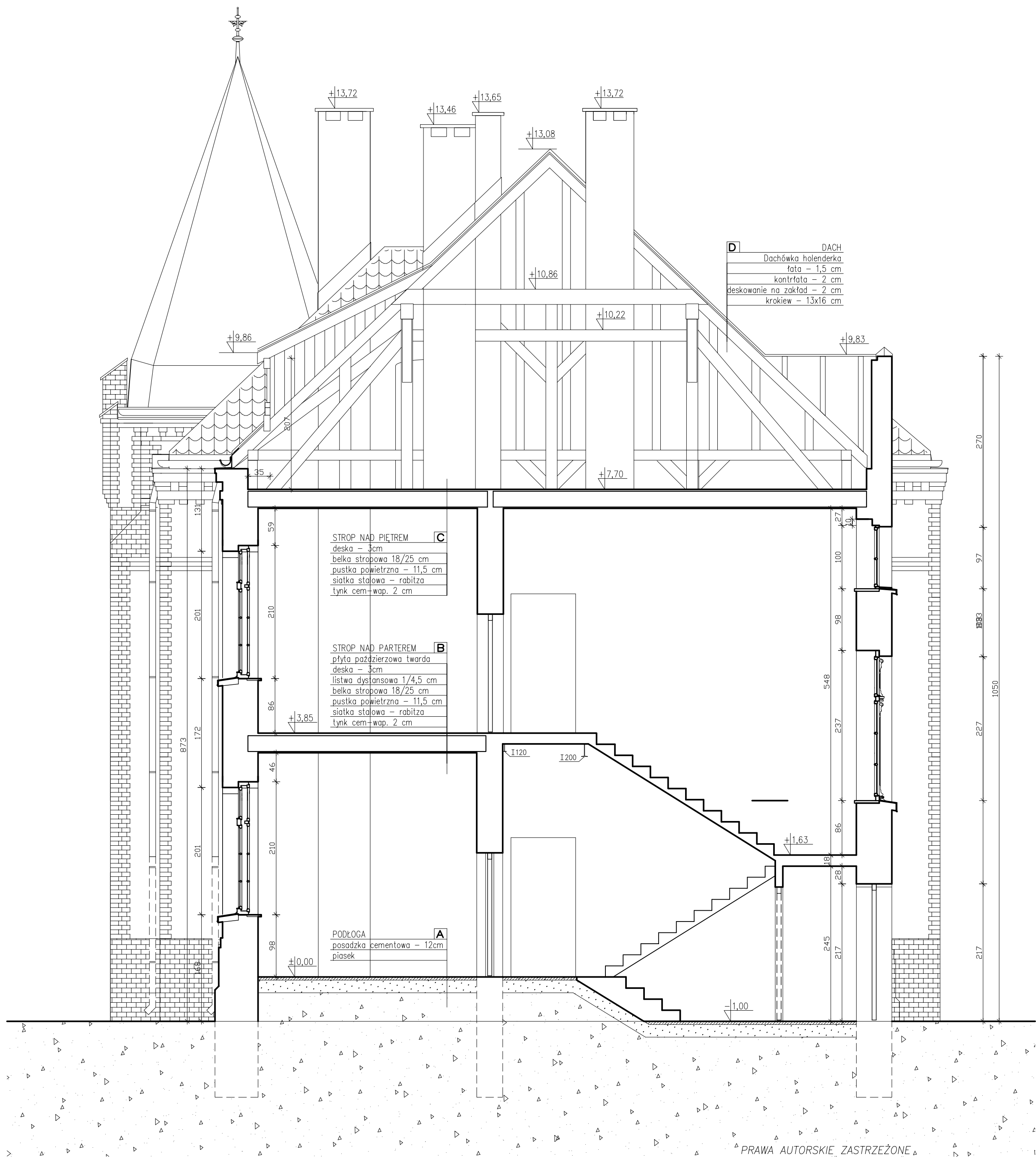
PRZEKRÓJ B-B SKALA 1:50
