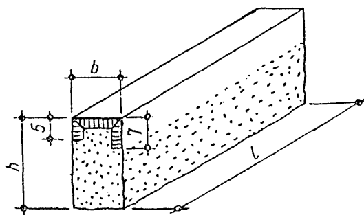
Rys. 5. Krawężnik drogowy rodzaju A
