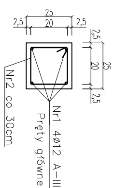
Szczegóły wieńca W-1 skala 1:20
