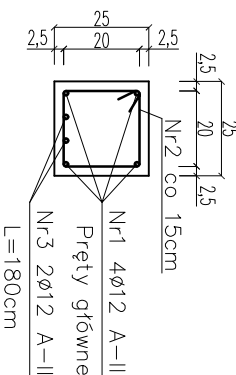
Szczegóły nadproża W-1: skala 1:20
